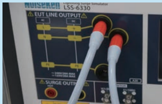
耦合部确认
