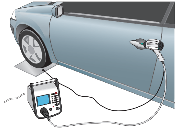
车辆内试验
