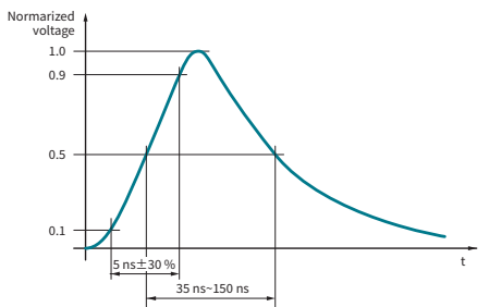
1 kΩ 负载时的脉冲波形
